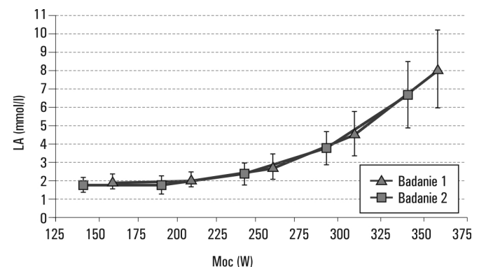
Rycina 2. Wykres zależności pomiędzy stężeniem mleczanu we krwi (LA) a obciążeniem wysiłkowym w teście progu beztlenowego w badaniu wyjściowym (Badanie 1) i po rocznym okresie treningu (Badanie 2) u badanych wioślarzy (n=30)
