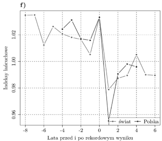
Rycina 2. Indeksy podstawowe oraz łańcuchowe w ujęciu analizowanych protokołów; a, c, e) indeksy jednopodstawowe; b, d, f) indeksy łańcuchowe
