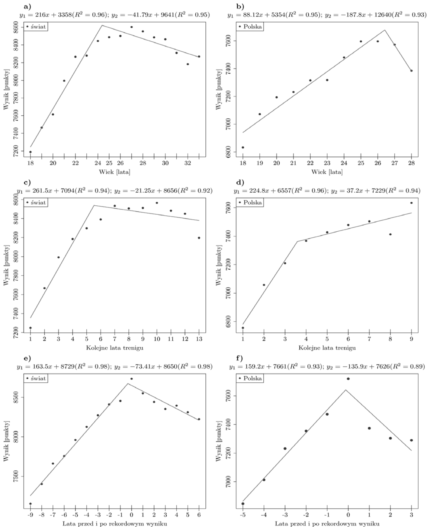
Rycina 1. Analiza trendów liniowych w ujęciu rozpatrywanych protokołów badawczych; a-b) protokół 1; c-d) protokół 2; e-f) protokół 3
