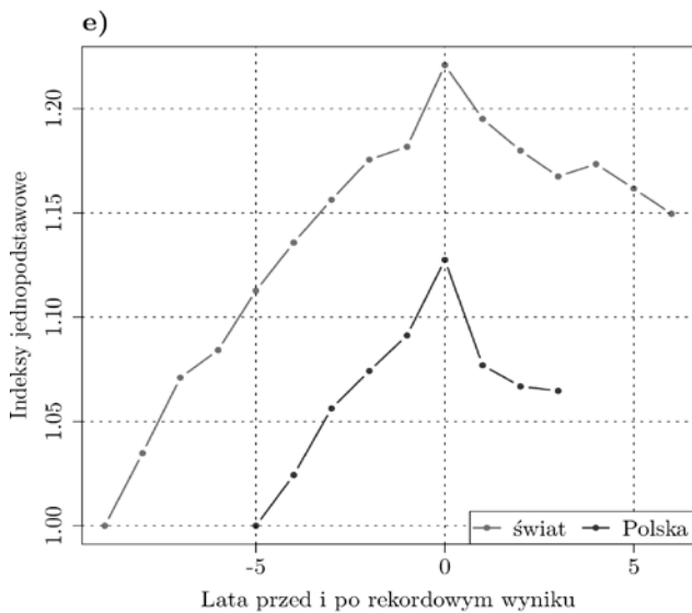
Rycina 2. Indeksy podstawowe oraz łańcuchowe w ujęciu analizowanych protokołów; a, c, e) indeksy jednopodstawowe; b, d, f) indeksy łańcuchowe
